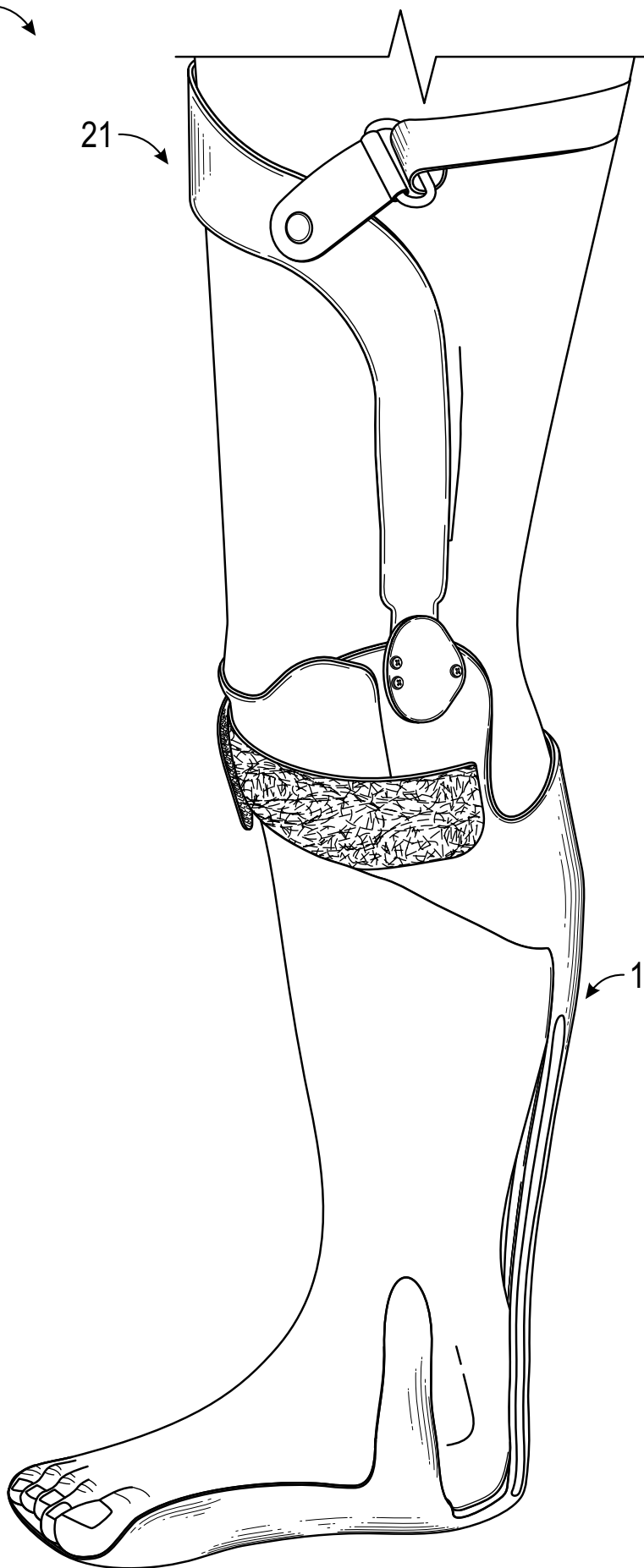
FIG. 9
