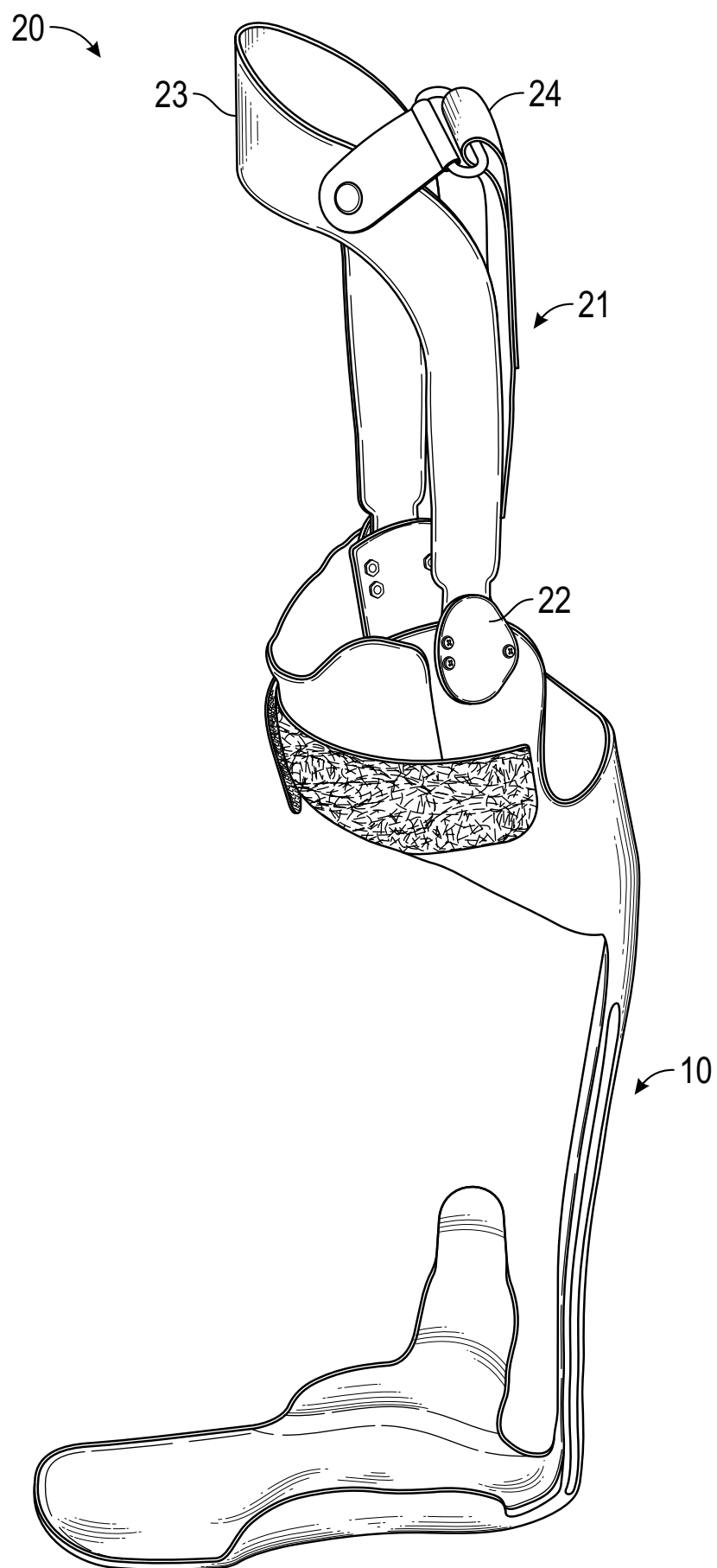
FIG. 7
